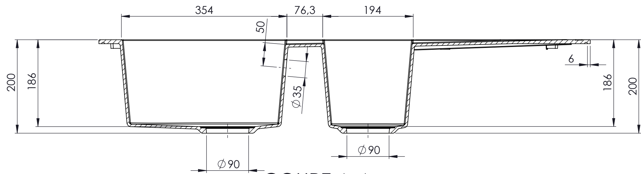
COUPE A-A
