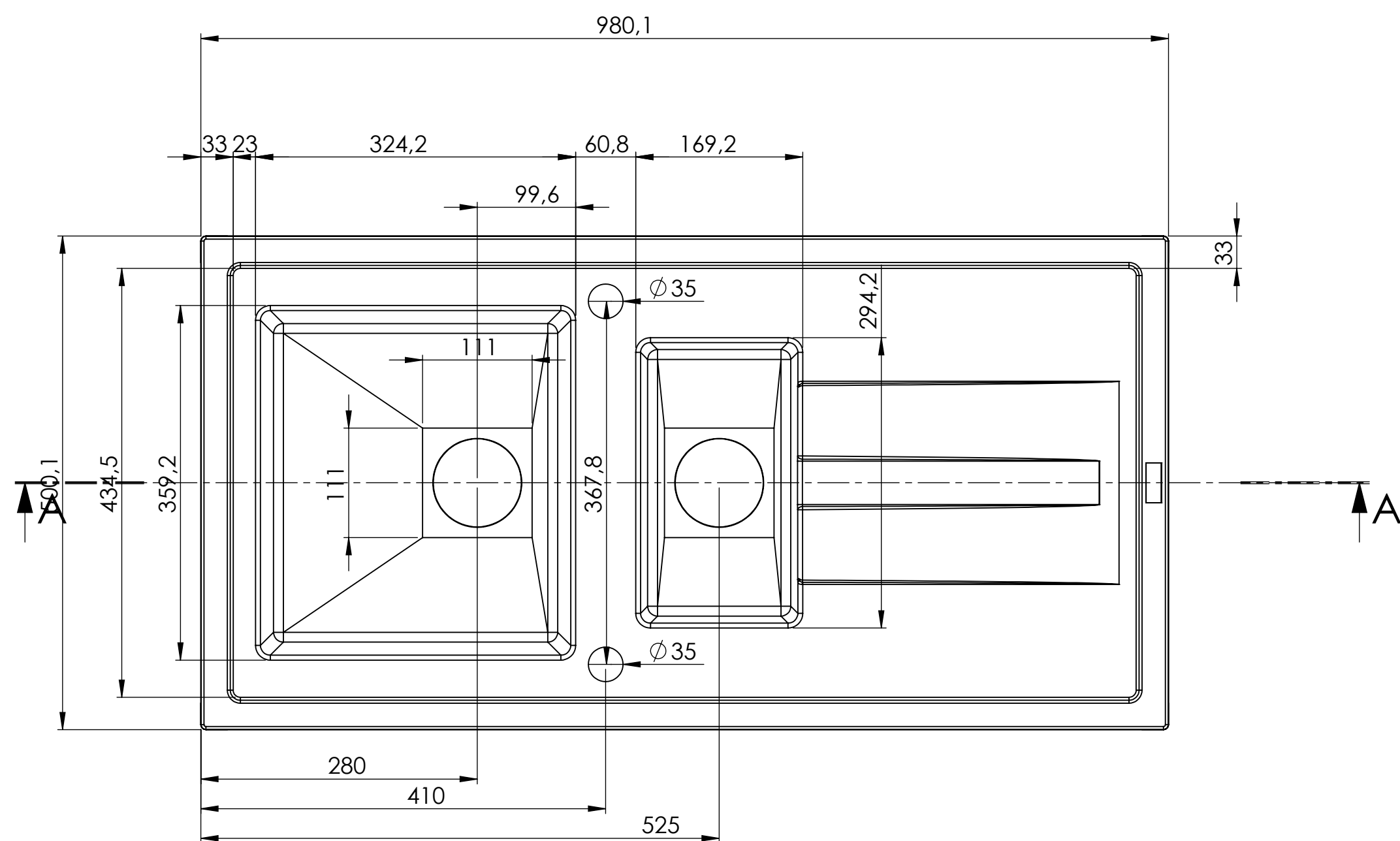
COUPE A-A
